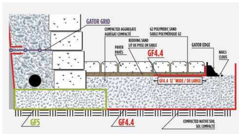
COUPE TYPE DE MUR GRAVITAIRE ET DE PAVÉ
