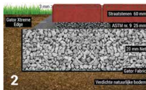
OPTIE 2 Open gegraven / waterdoorlatend
